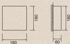
DIVETRO 18 LED 17W - 230VAC - 3000K C€ weight - 0,75 kg
