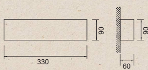
DIVETRO 33 LED 9W - 230VAC - 3000K C€ weight - 0,75 kg
